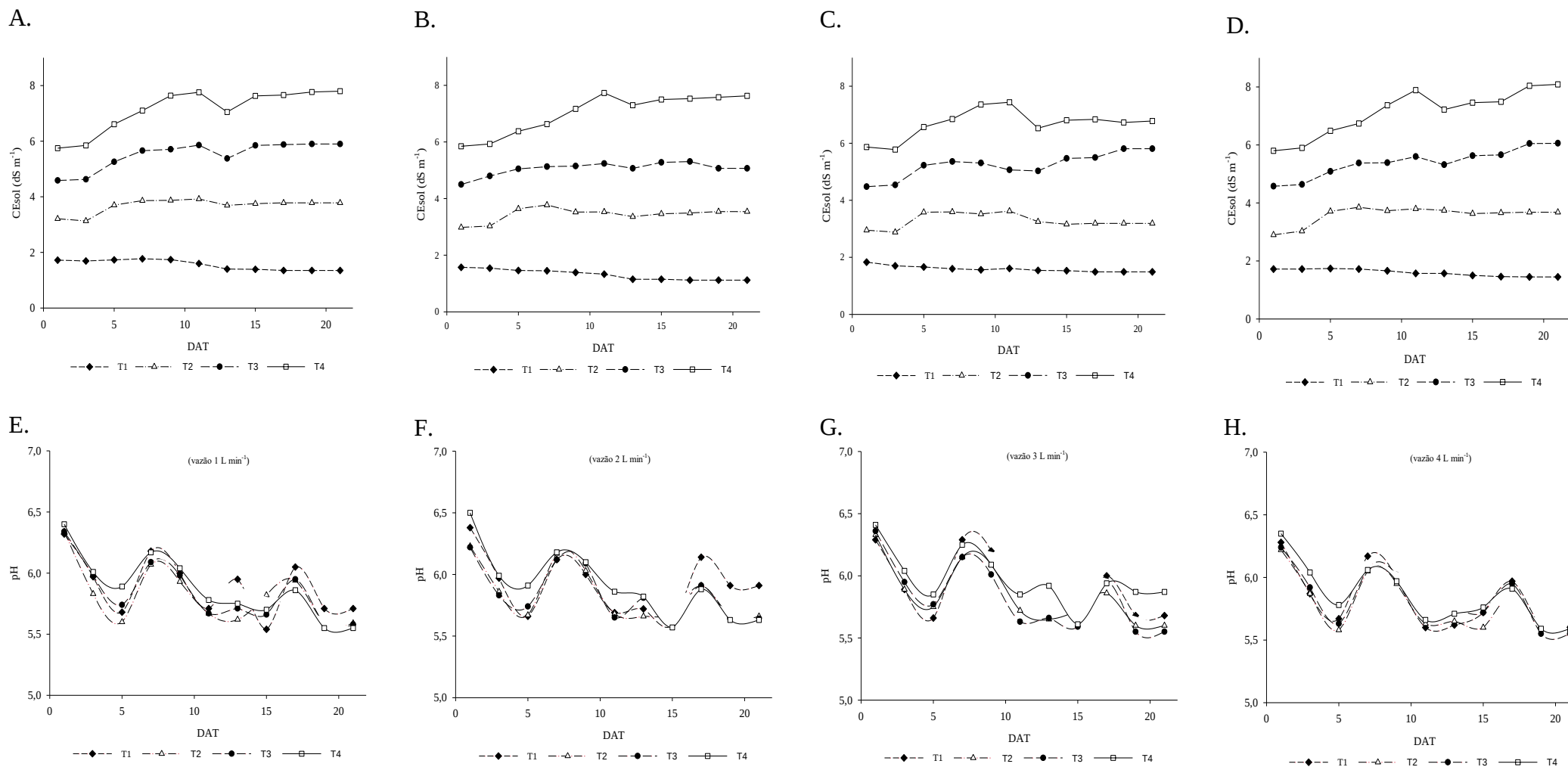
Figura 13. Valores médios de CEsol (A) e de pH (E) da solução nutritiva na vazão de 1 L min -1 ; CEsol (B) e de pH (F) na vazão de 2 L min -1 ; CEsol (C) e de pH (G) na vazão 3 L min -1 ; CEsol (D) e de pH (H) na vazão 4 L min -1 ao longo do ciclo de cultivo do Coentro, cultivar “verdão”, experimento II, água cálcica.
