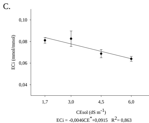
Figura 20. Eficiência instantânea de carboxilação ( EC_i ) do coentro cultivar Verdão, submetido a diferentes níveis de salinidade e vazões da solução nutritiva, preparada em águas salinizadas com NaCl (A), \text{CaCl}_2 (B) e uma mistura de sais na proporção 2:1:1 (NaCl : \text{CaCl}_2 \cdot 2\text{H}_2\text{O} : \text{MgCl}_2 \cdot 6\text{H}_2\text{O} ) (C), em Recife-PE, *: regressão significativa a 5% de probabilidade; **: regressão significativa a 1% de probabilidade.
