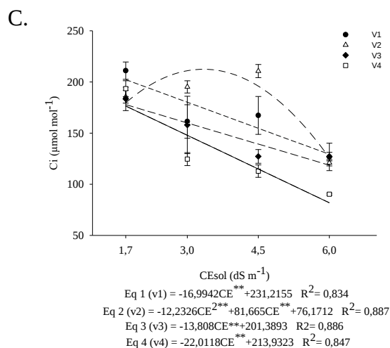
Figura 16. Concentração interna de \text{CO}_2 do coentro cultivar Verdão, submetido a diferentes níveis de salinidade e vazões da solução nutritiva, preparada em águas salinizadas com NaCl (A), \text{CaCl}_2 (B) e uma mistura de sais na proporção 2:1:1 (NaCl : \text{CaCl}_2 \cdot 2\text{H}_2\text{O} : \text{MgCl}_2 \cdot 6\text{H}_2\text{O} ) (C), em Recife-PE, *: regressão significativa a 5% de probabilidade; **: regressão significativa a 1% de probabilidade.
