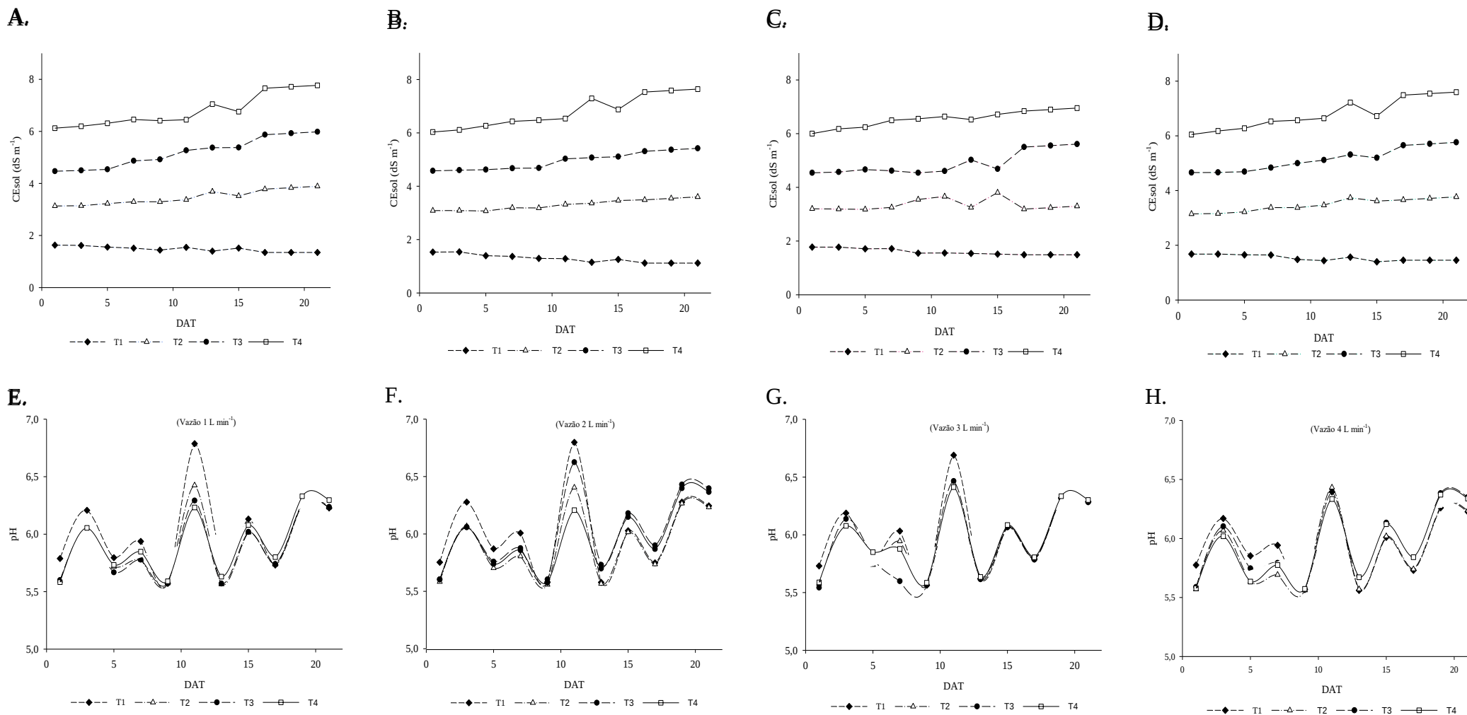
Figura 14. Valores médios de CEsol (A) e de pH (E) da solução nutritiva na vazão de 1 \text{L min}^{-1} ; CEsol (B) e de pH (F) na vazão de 2 \text{L min}^{-1} ; CEsol (C) e de pH (G) na vazão 3 \text{L min}^{-1} ; CEsol (D) e de pH (H) na vazão 4 \text{L min}^{-1} ao longo do ciclo de cultivo do Coentro, cultivar “verdão”, experimento III, água mista.
