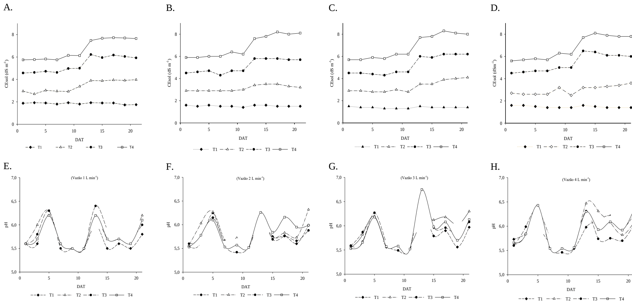
Figura 12. Valores médios de CEsol (A) e de pH (E) da solução nutritiva na vazão de 1 \text{L min}^{-1} ; CEsol (B) e de pH (F) na vazão de 2 \text{L min}^{-1} ; CEsol (C) e de pH (G) na vazão 3 \text{L min}^{-1} ; CEsol (D) e de pH (H) na vazão 4 \text{L min}^{-1} ao longo do ciclo de cultivo do Coentro, cultivar “verdão”, experimento I, água sódica.
