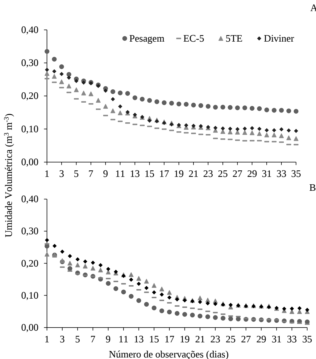
Figura 2. Curvas de secagem dos solos estudados em função dos valores de umidade estimada pelos sensores EC-5, 5TE e Diviner e a umidade gravimétrica (pesagem) convertida em umidade volumétrica; (A) Solo de textura franco argilo arenosa; (B) Solo de textura areia.
