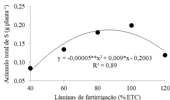
Figura 15 - Acúmulo total de enxofre (S) em função das lâminas de fertirrigação aplicadas (A) e dos tipos de aplicação da fertirrigação (B). Carpina-PE, 2022. Letras diferentes indicam diferenças significativas entre os tipos de aplicação da fertirrigação (pulsada e contínua) pelo teste de Scott Knott ( p < 0,05 ).
