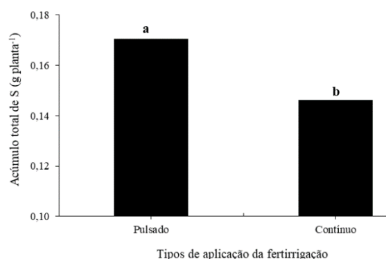
Figura 15 - Acúmulo total de enxofre (S) em função das lâminas de fertirrigação aplicadas (A) e dos tipos de aplicação da fertirrigação (B). Carpina-PE, 2022. Letras diferentes indicam diferenças significativas entre os tipos de aplicação da fertirrigação (pulsada e contínua) pelo teste de Scott Knott ( p < 0,05 ).
