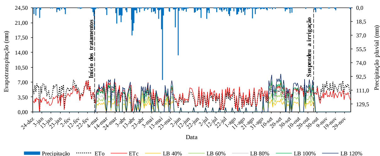
Figura 1. Valores de precipitação, evapotranspiração de referência (ET o ), evapotranspiração da cultura (ET c ), e lâmina bruta aplicada nos tratamentos de 40% (LB 40%), 60% (LB 60%) 80% (LB 80%), 100% (LB 100%) e 120% (LB 120%) da ET c na cultura da cana-de-açúcar. Carpina - PE, 2021.
